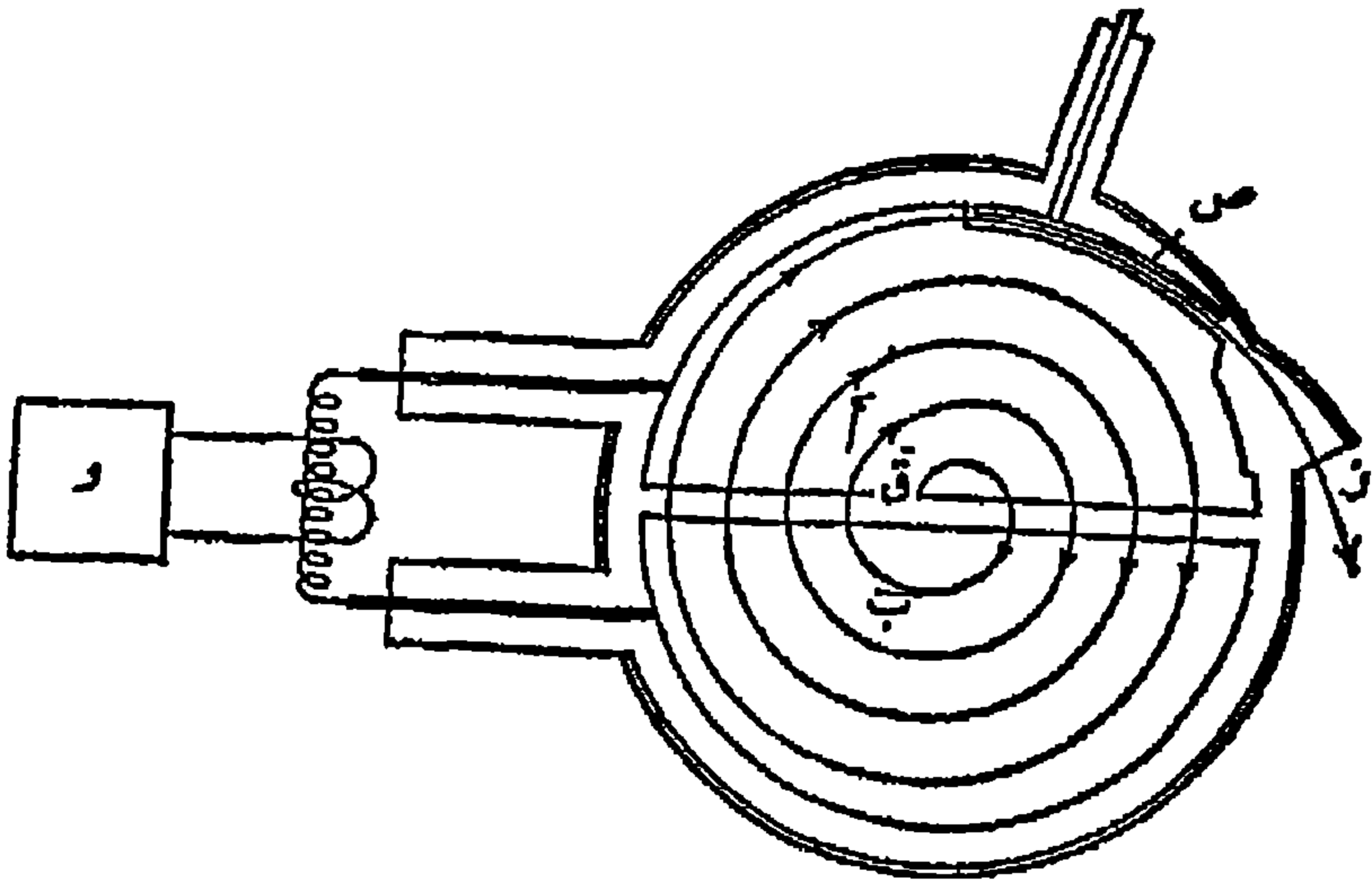
الشكل ٥ . - السيكلوترون
