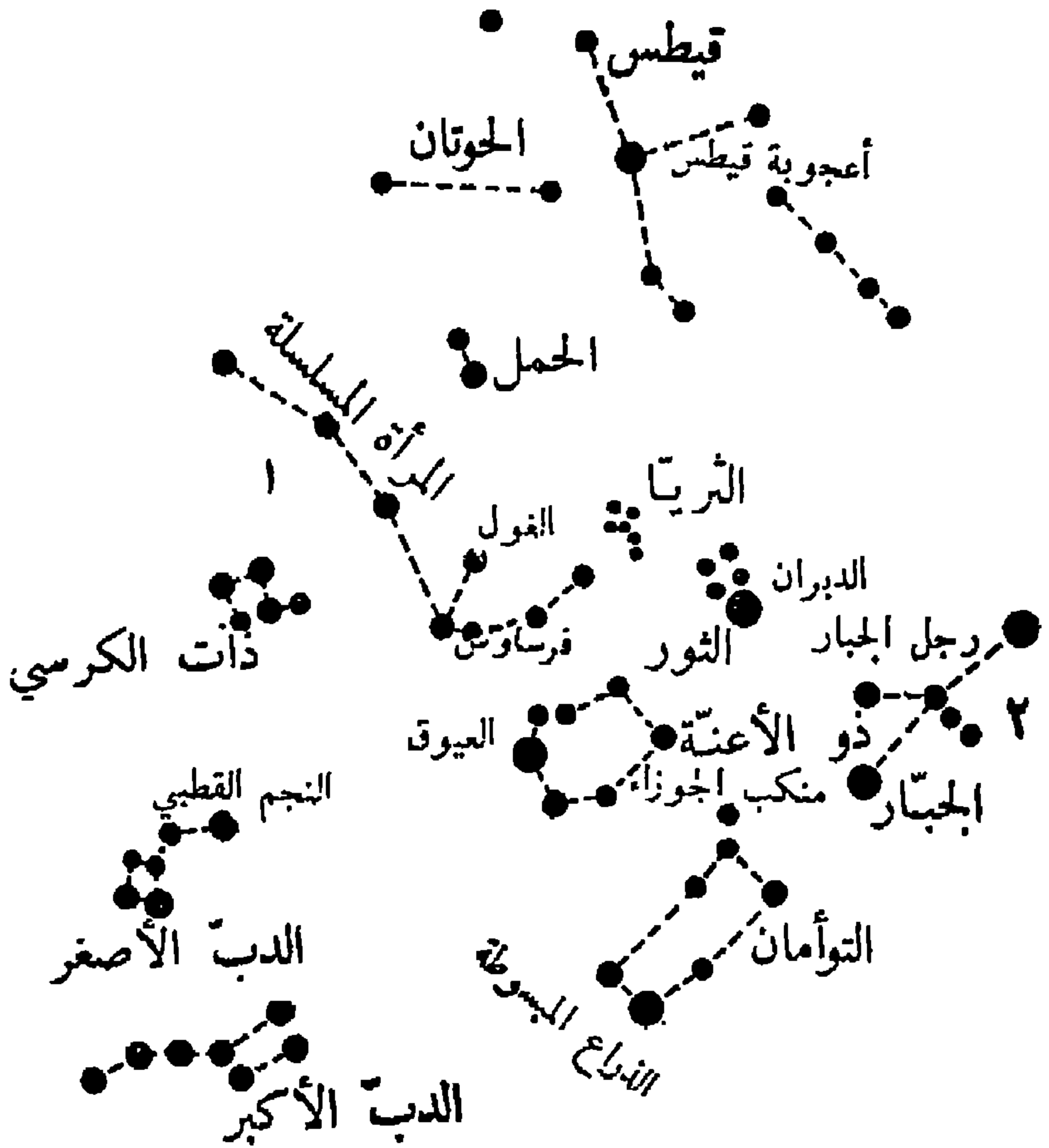
الشكل ٧ . - موقع مجرة المرأة المسلسلة (١٠+) وسديم الجبار (٢) في السماء الشمالية
