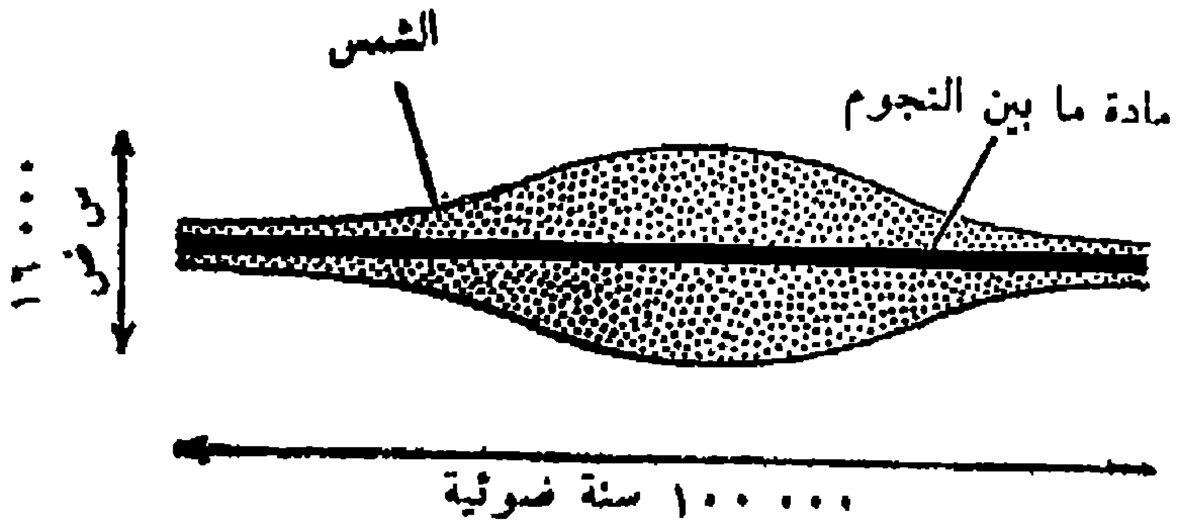
الشكل ٨ - المجرة
