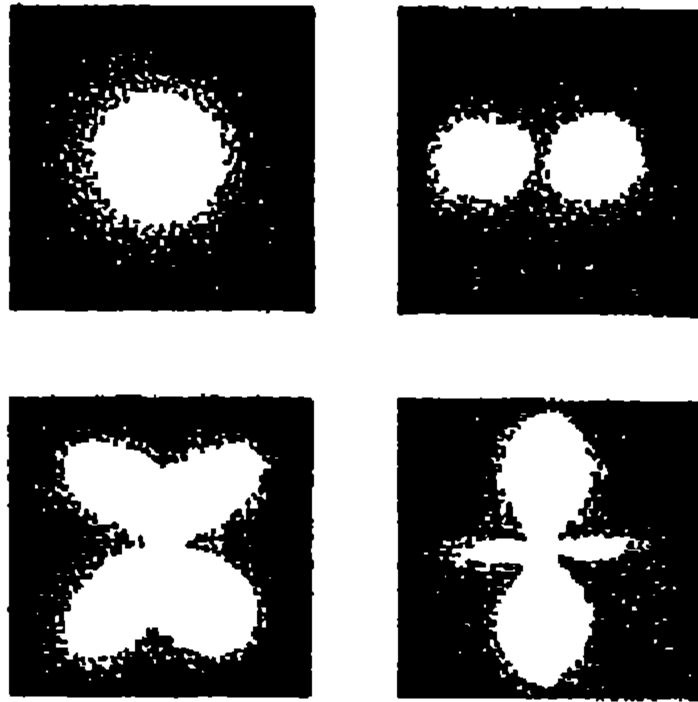
الشكل ٣ . - الذرة حسب الميكانيكا التمرجية
